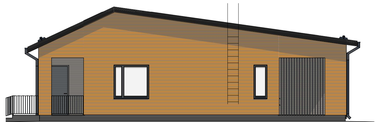
JULKISIVU KOILLISEEN
